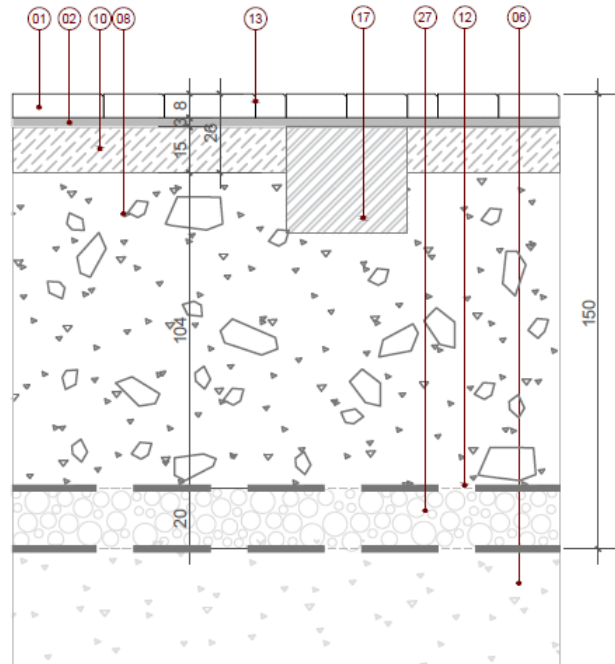
DETALL P4 SOL ESTRUCTURAL ZONA VIANANTS PAVIMENT PEDRA NATURAL GRANÍTICA 8 CM SENSE LLOSA FORMIGÓ
